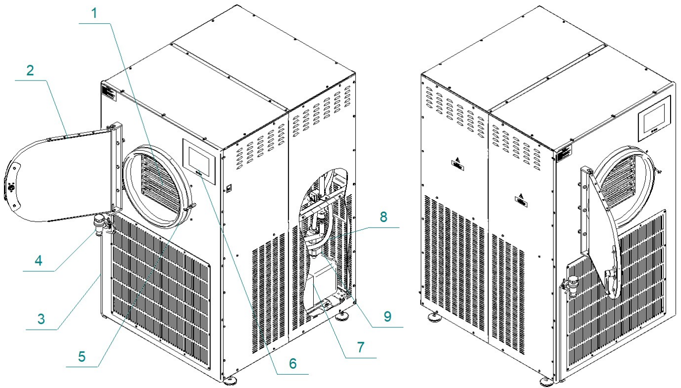
Рис. 1. Лиофильная сушильная камера ЛФ-16, ЛФ-16П, ЛФ-25, ЛФ-25П
